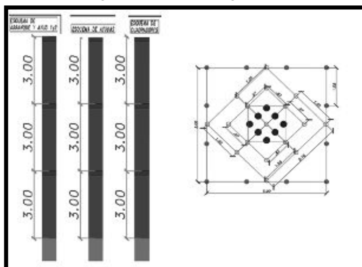
Figura 33: Diseño de carguío VCR.
