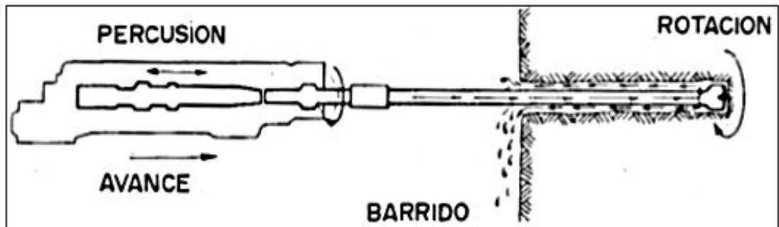
Figura N° 8 Máquina perforadora.
