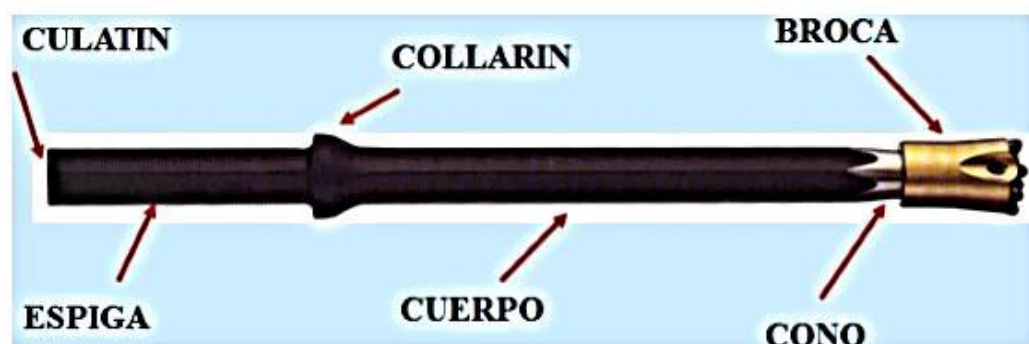
Figura N° 11 Varillaje Cónico
