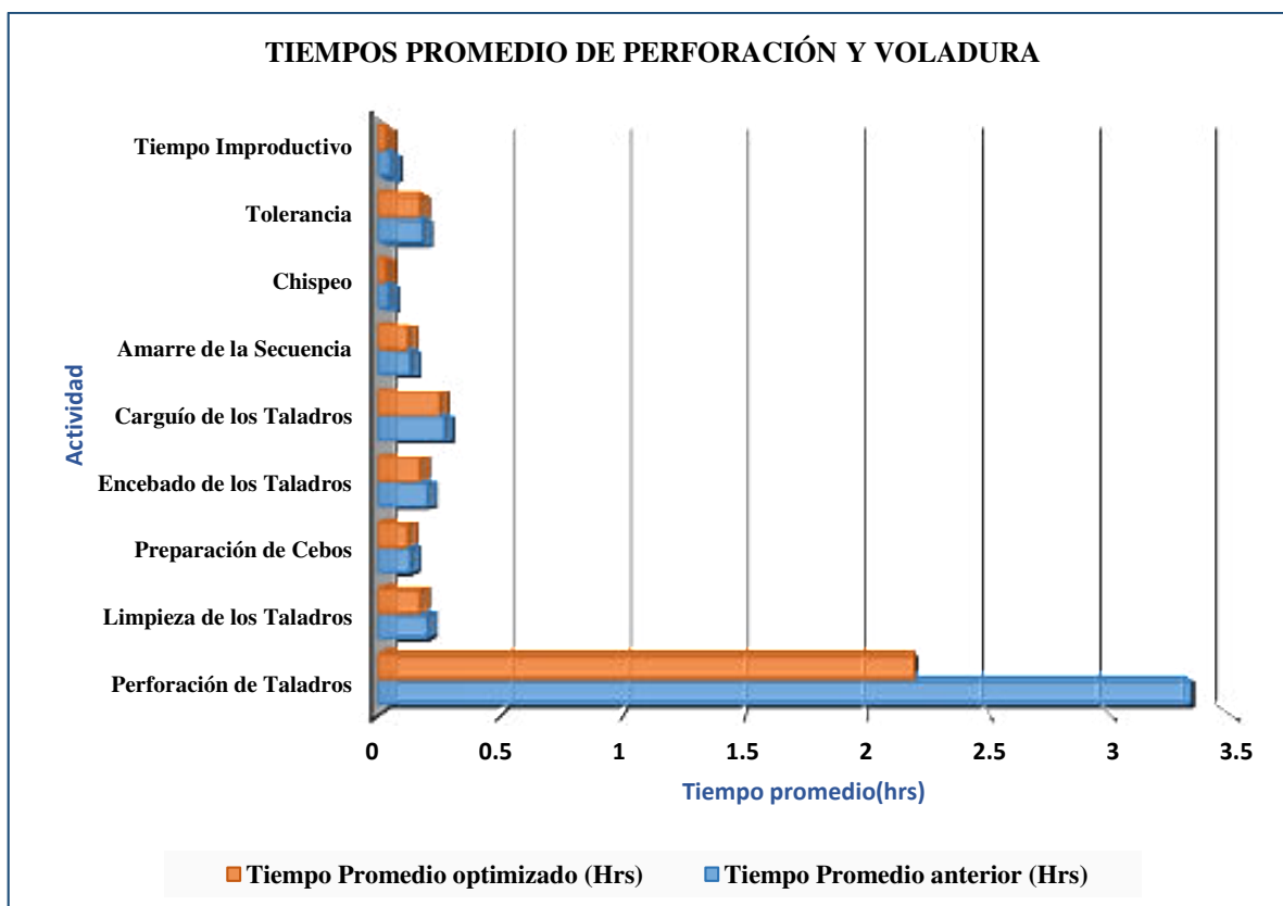
Figura N° 29 Tiempos promedio de perforación y voladura
