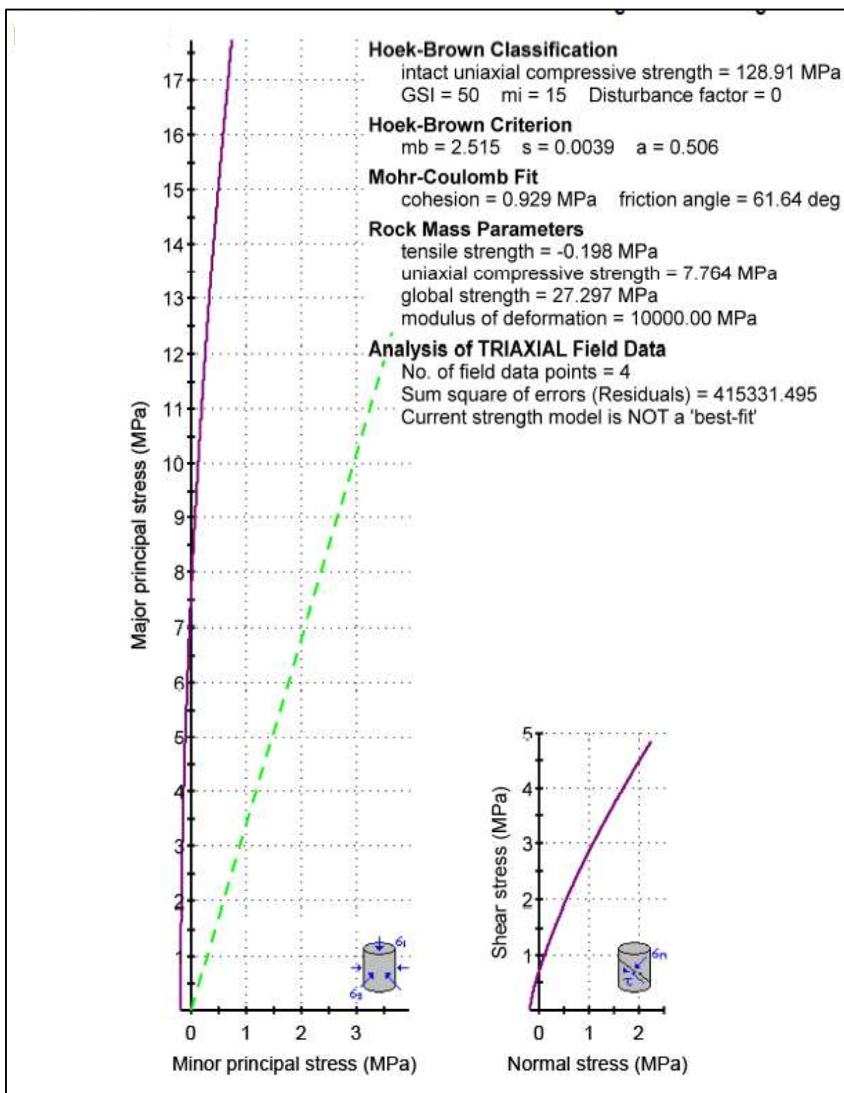
Figura 39 — Resultado del software de rocdata del comportamiento geomecánico elasto frágil de la muestra arenisca.
