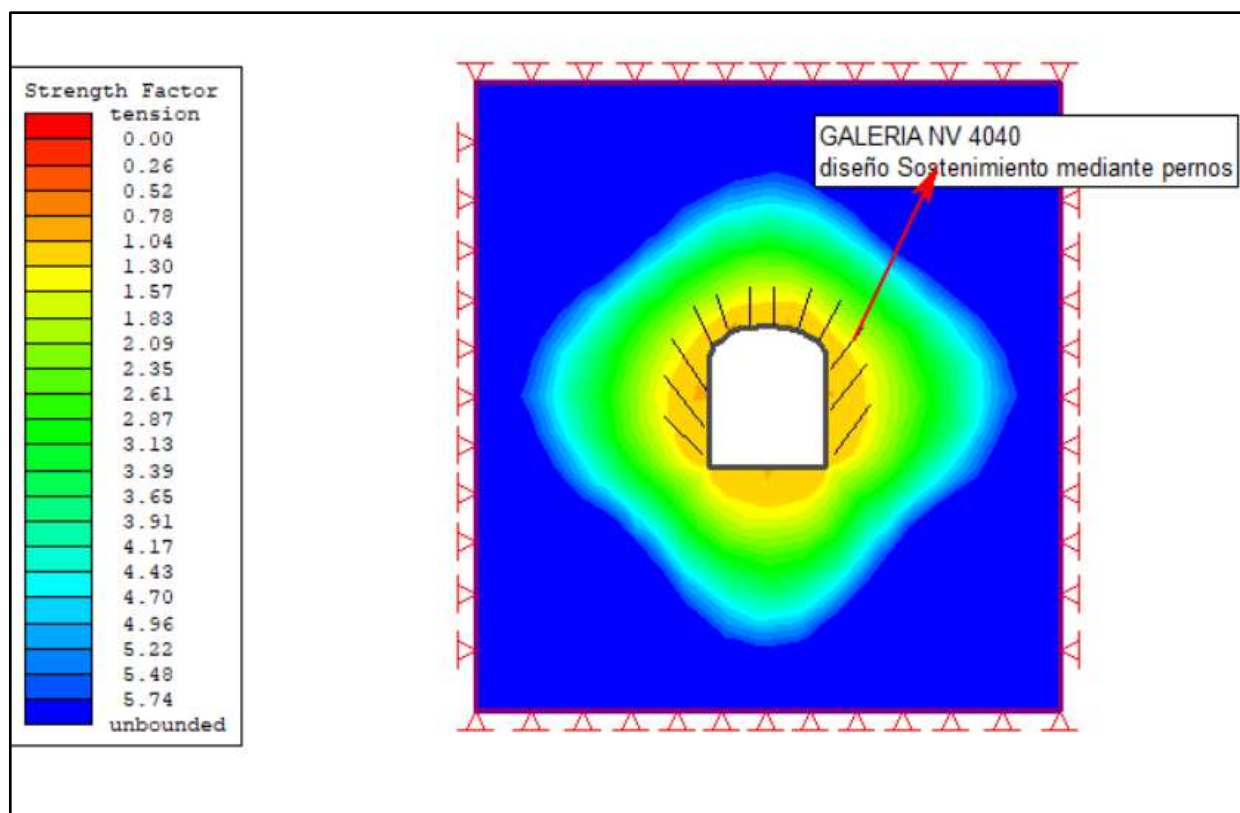
Figura 20 — Diseño del tipo de sostenimiento con pernos de anclaje de la galería nivel 4040
