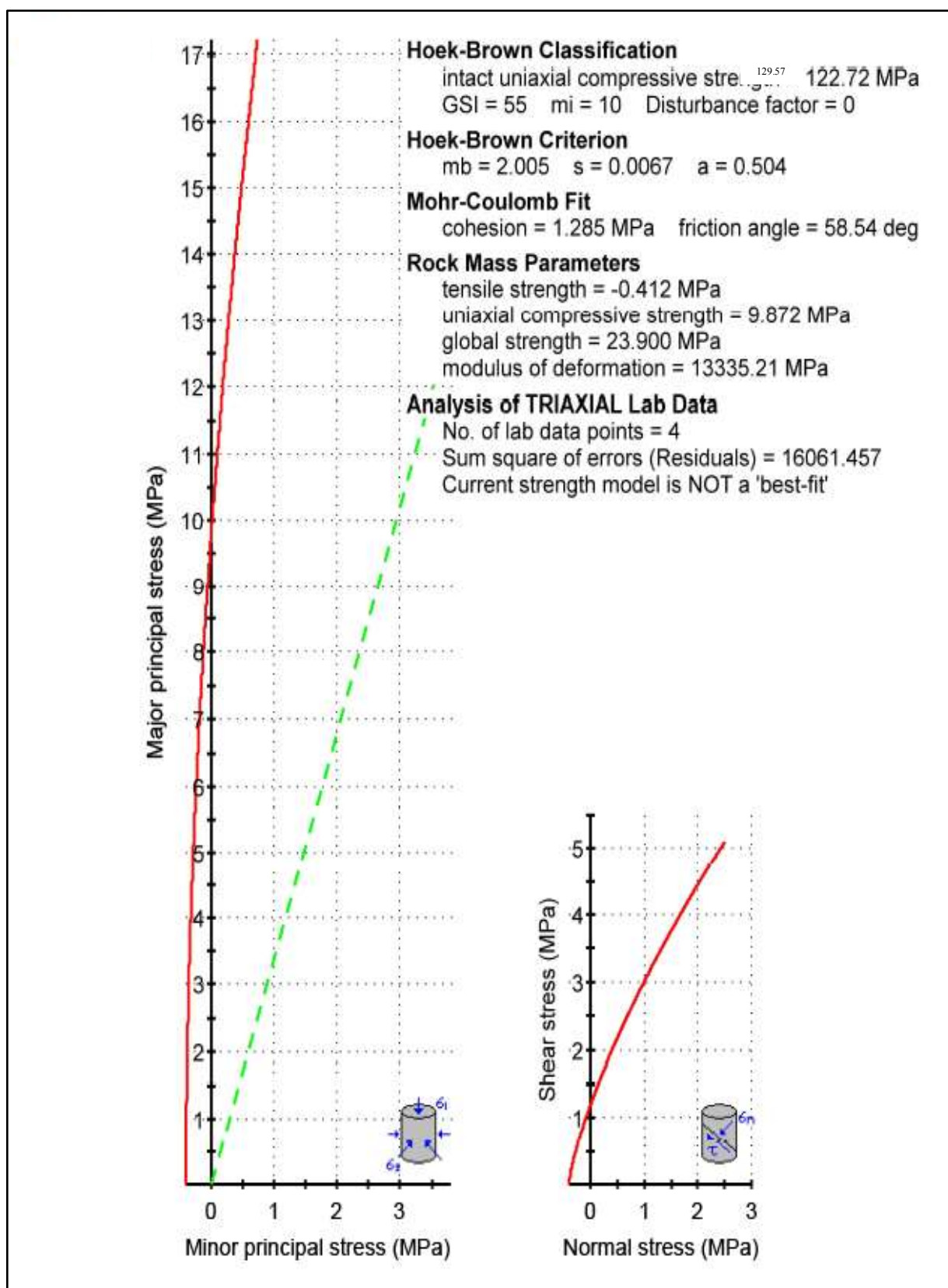
Figura 38 — Resultado del software rocdata del comportamiento geomecánico elasto frágil de la muestra caliza.
