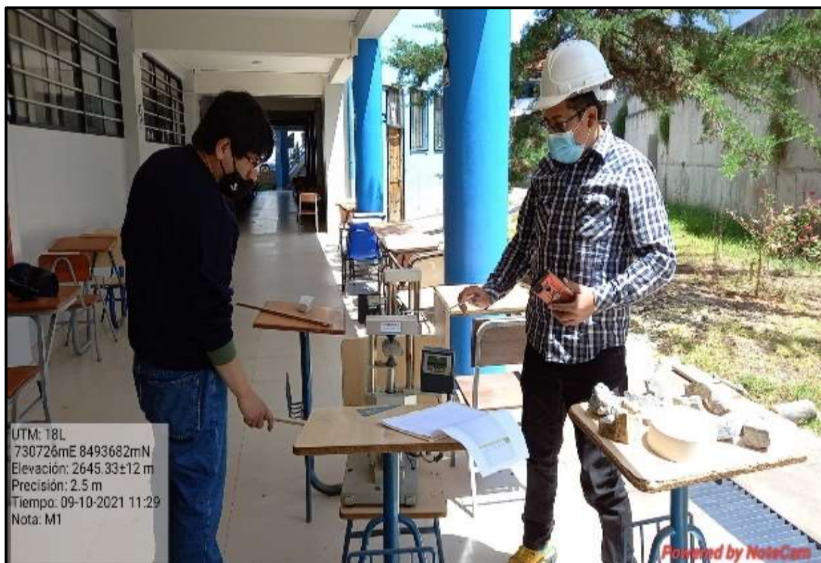
Figura 69 — Realización de ensayos con el uso de equipo de carga puntual
