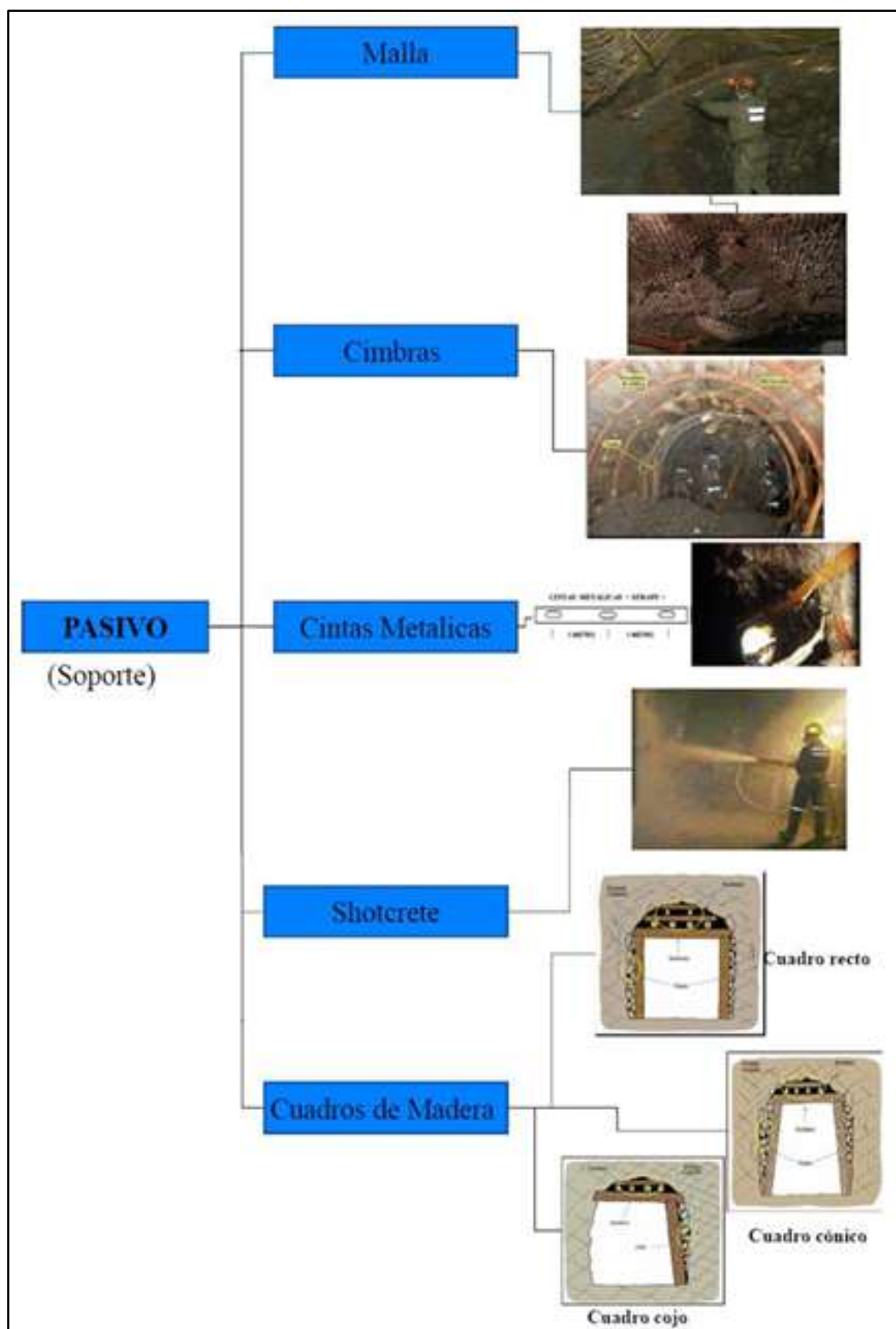
Figura 5 — Tipos de sostenimiento pasivo
