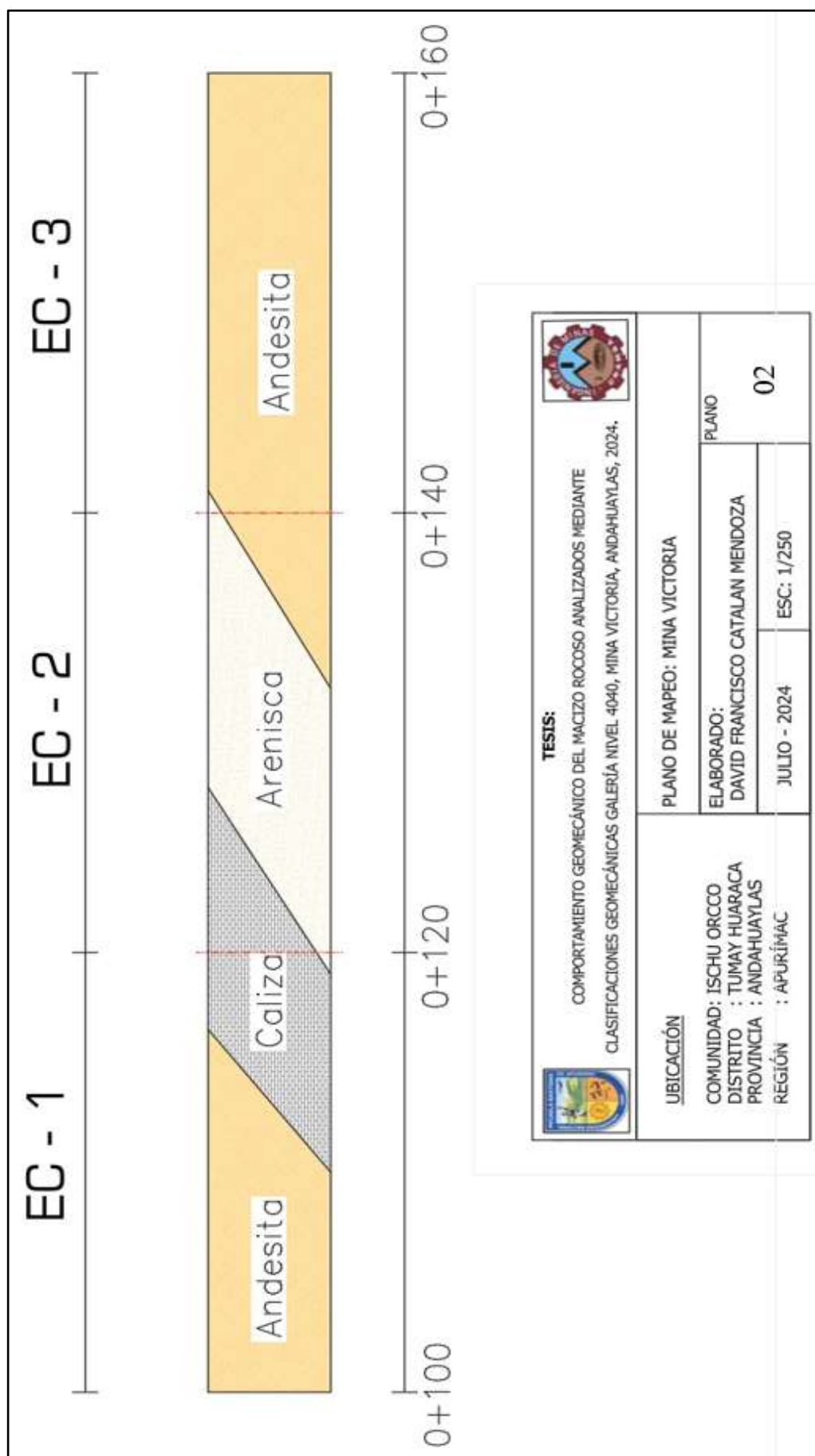
Figura 74 — Mapeo geomecánico de las rocas de la mina la Victoria
