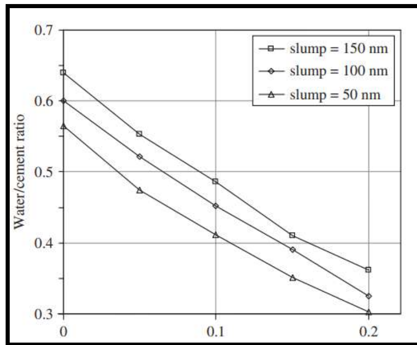
Figura 5 — Trabajabilidad del hormigón con látex
