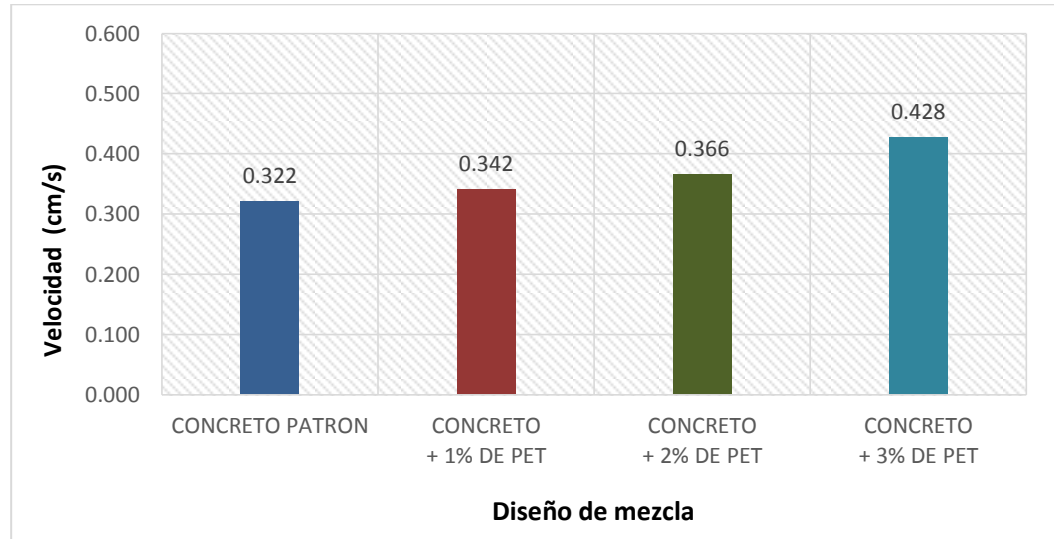
Figura 22 — Permeabilidad del concreto permeable
