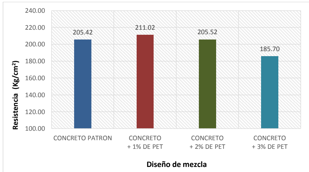
Figura 19 — Resistencia a la compresión del concreto permeable a 28 días
