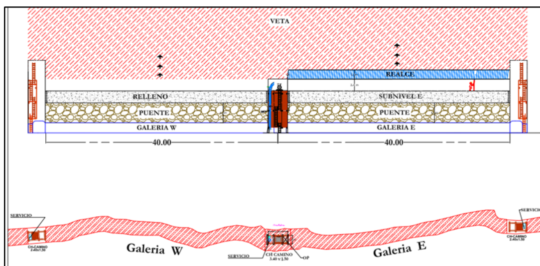
Figura 15 Corte Relleno Convencional CRC:
