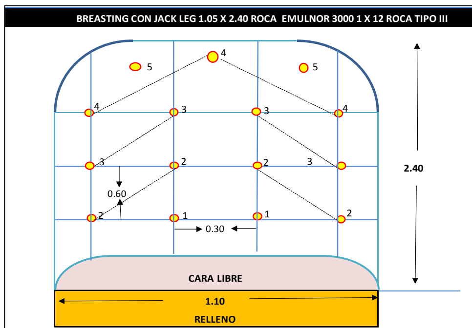
Figura 16. BRESTING CON JACK LEG
