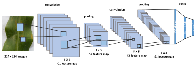
Fig. 2. Una arquitectura de CNN
