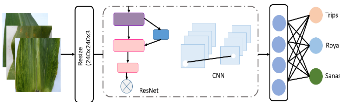
Fig. 3. Una arquitectura ResNet
