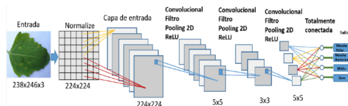
Fig. 3. Arquitectura de Modelo de Red Neuronal Convolucional.
