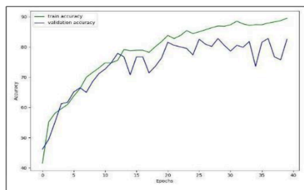
Fig. 5. Análisis de Precisión del Modelo Propuesto
