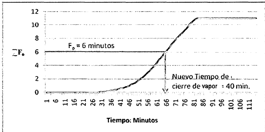
FIGURA 11: CURVA DE LETALIDAD TERMICA
