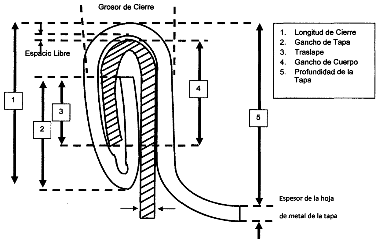
FIGURA N°5: DENOMINACIONES ESTÁNDARES PARA LOS COMPONENTES DE SELLO DOBLE
