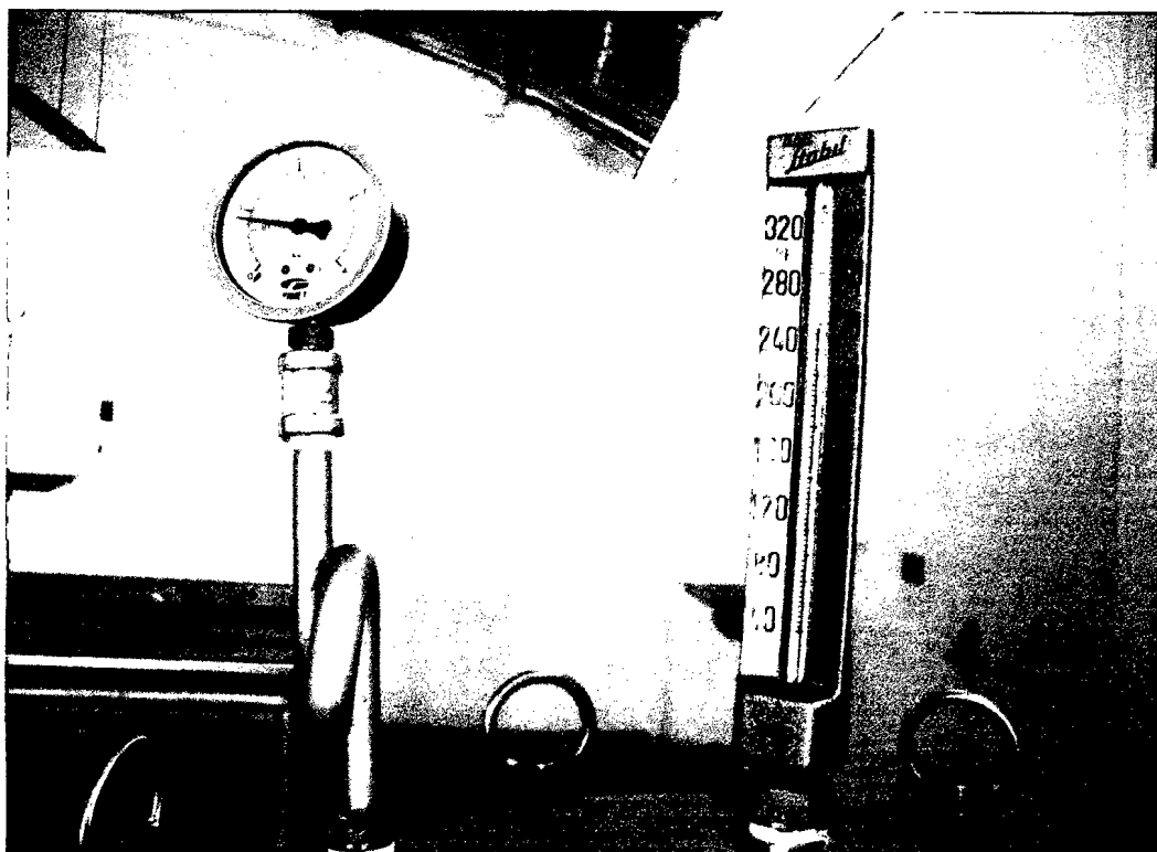
Foto N° 15: Instrumentos de control de temperatura y presión de autoclaves
