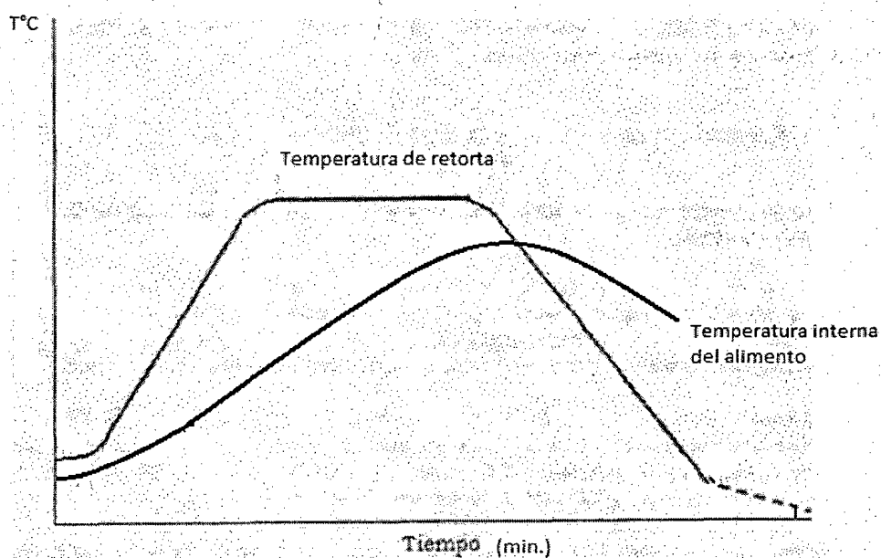
FIGURA 6: CURVA DE TEMPERATURA INTERNA DEL ALIMENTO Y TEMPERATURA DE RETORTA (MÉTODO GENERAL)
