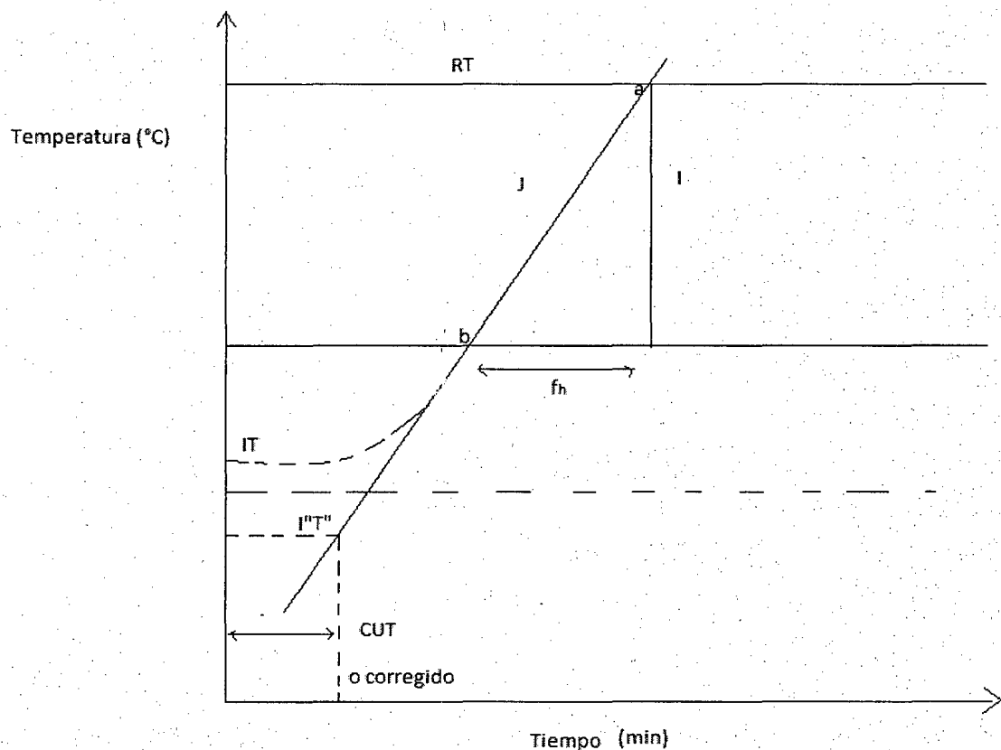
FIGURA 7: GRÁFICO DEL MÉTODO DE LA FORMULA DE BALL
