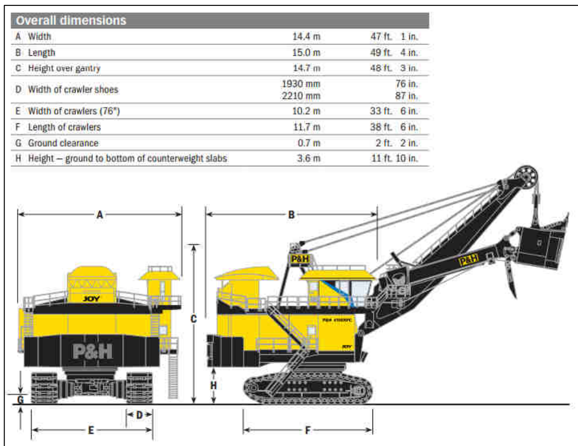
FIGURA 2- 43. Dimensiones de P&H4100XPC
