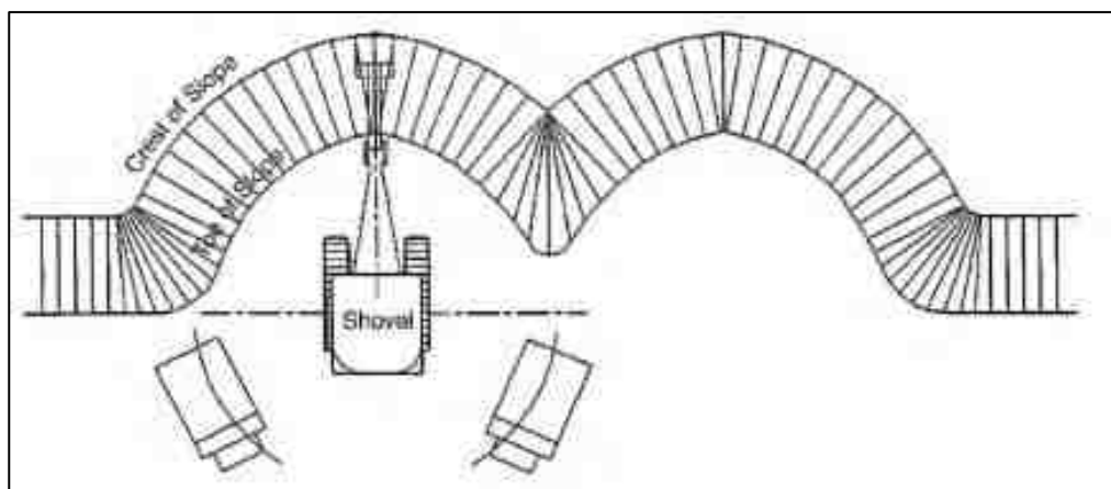
FIGURA 2- 28. Movimiento de Pala en corte Frontal
