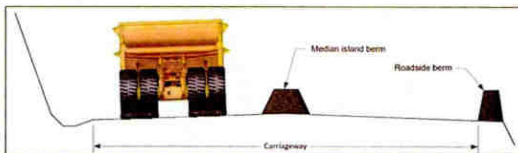
FIGURA 3-17. Ubicación de las bermas de seguridad para vías. Fuente: RJ Thompson (2015).
