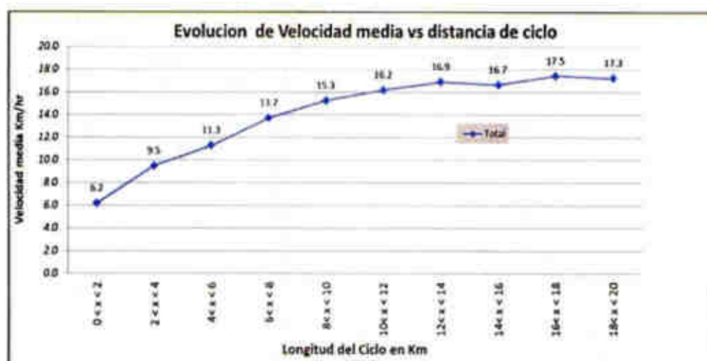
FIGURA 5-10. Evolución de la Velocidad Media vs Distancia del Ciclo.
