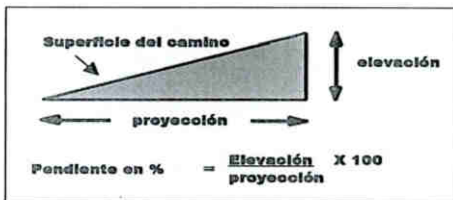
FIGURA 3-11. Pendiente de una vía de acarreo.
